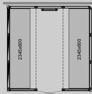
PANACEA 2525 2B Maße: 2525 x 2525 x 2090 mm
