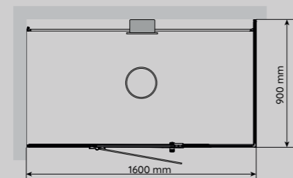
VISTA 160 RECHTS Maße: T 900 x B 1600 mm
