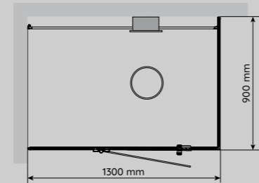
VISTA 130 RECHTS Maße: T 900 x B 1300 mm
