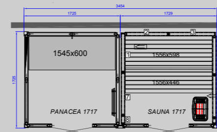
TWIN PANACEA 1717 Maße: T 1725 x B 3454 mm
