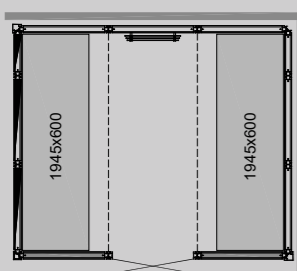
PANACEA 2521 2B Maße: 2525 x 2125 x 2090 mm
