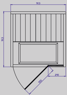
TYLÖSAND T-810 Maße: T 913 x B 913 mm
