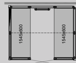
PANACEA 2117 2B Maße: 2125 x 1725 x 2090 mm
